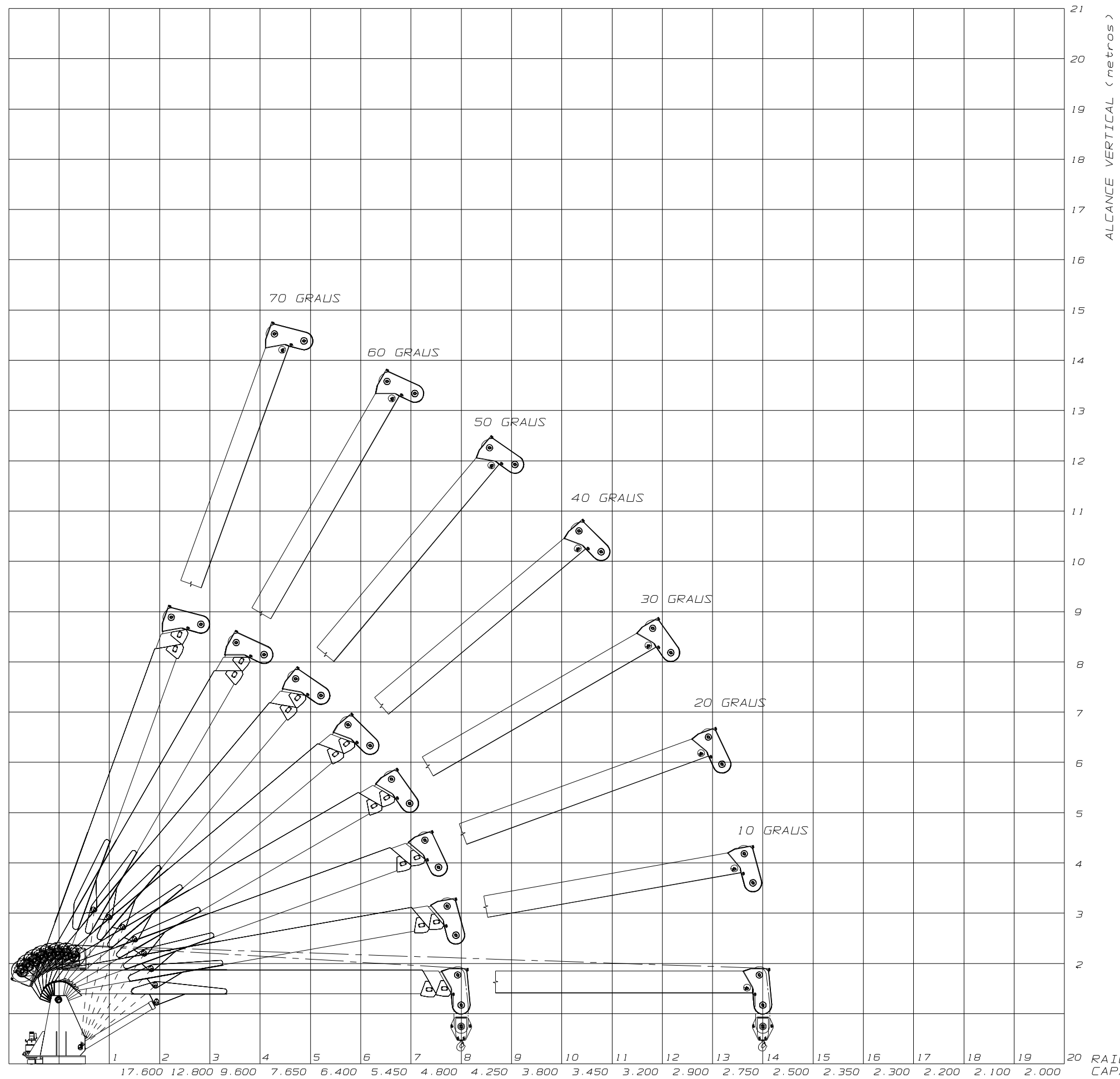
DIAGRAMA DE ALCANCE / ALCANCE GUINDASTE TELESCOPICO DE PRVISOES MODELO: EP - 6011
