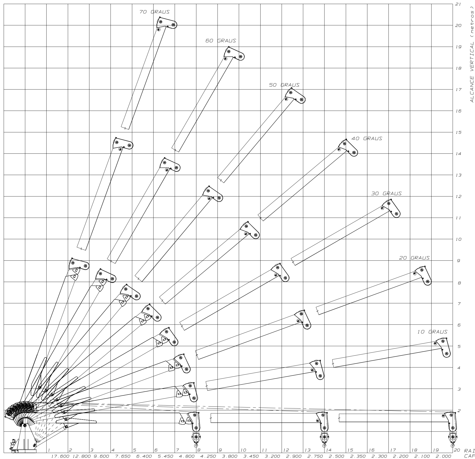
DIAGRAMA DE ALCANCE / ALCANCE GUINDASTE TELESCOPICO DE PRVISOES MODELO: EP - 6022
